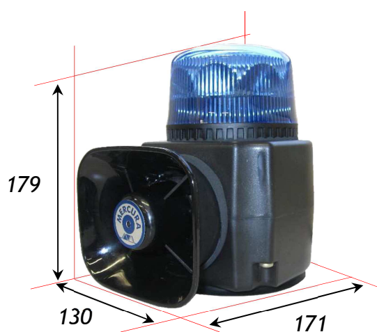
Version support magnétique Poids : 2,4 Kg
